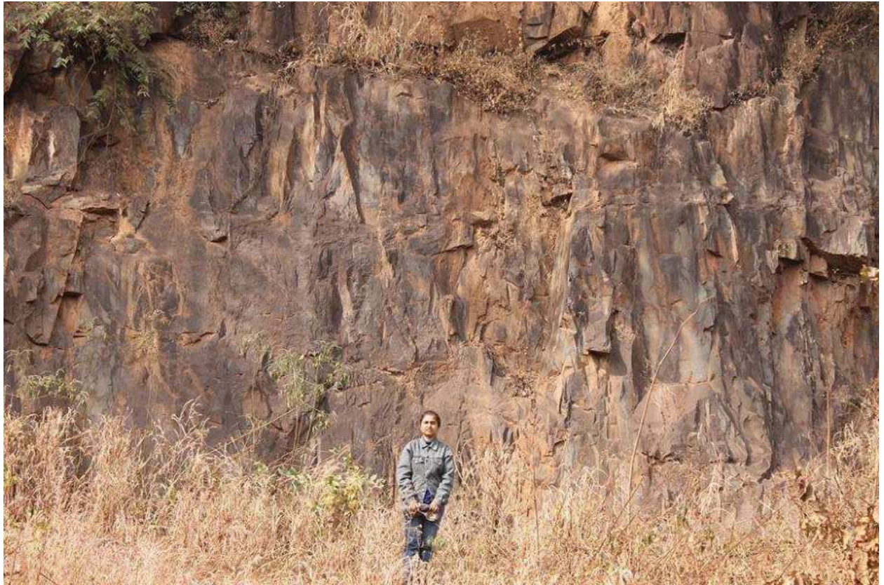
IOG, Columnar Basalt, Koirā area
